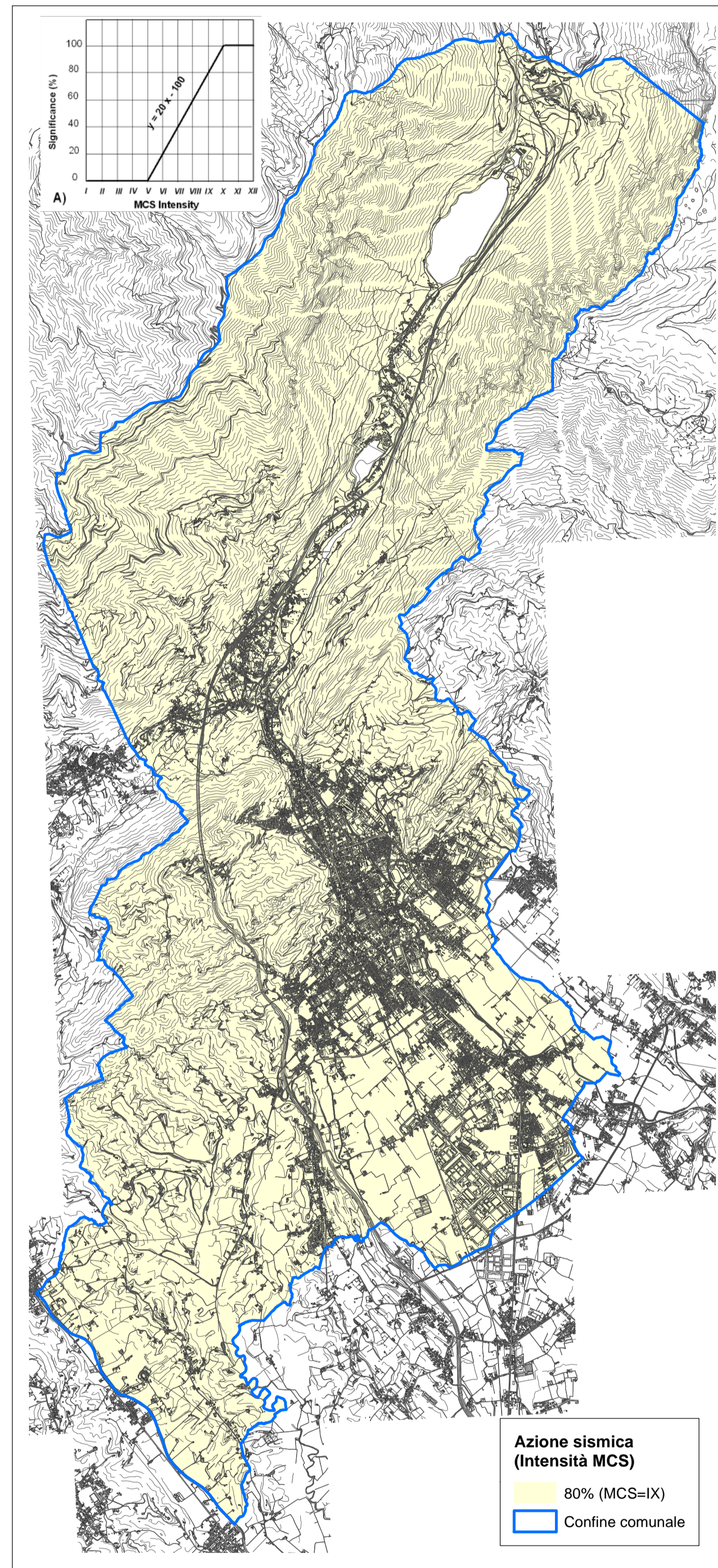
Parametro C: Sismicità
