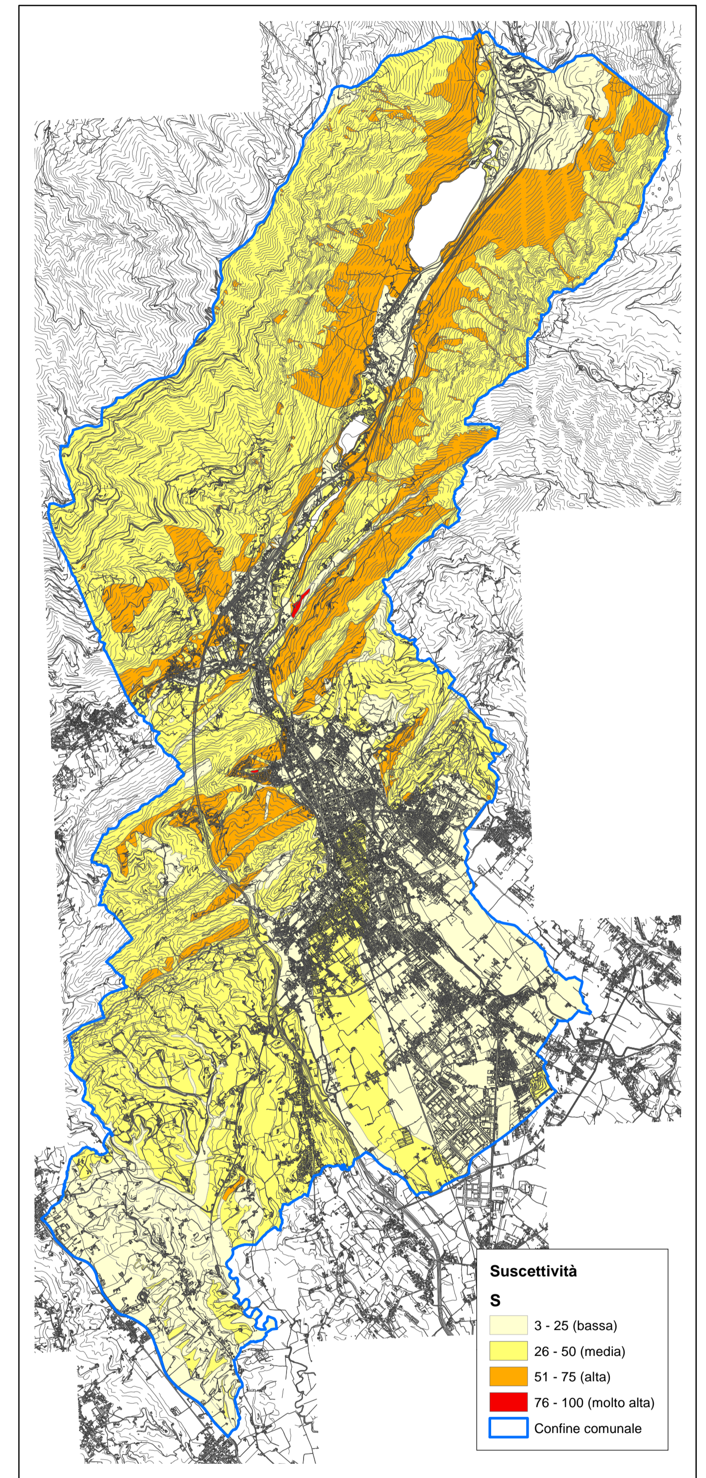
Carta della suscettibilità alle frane sismo-indotte
