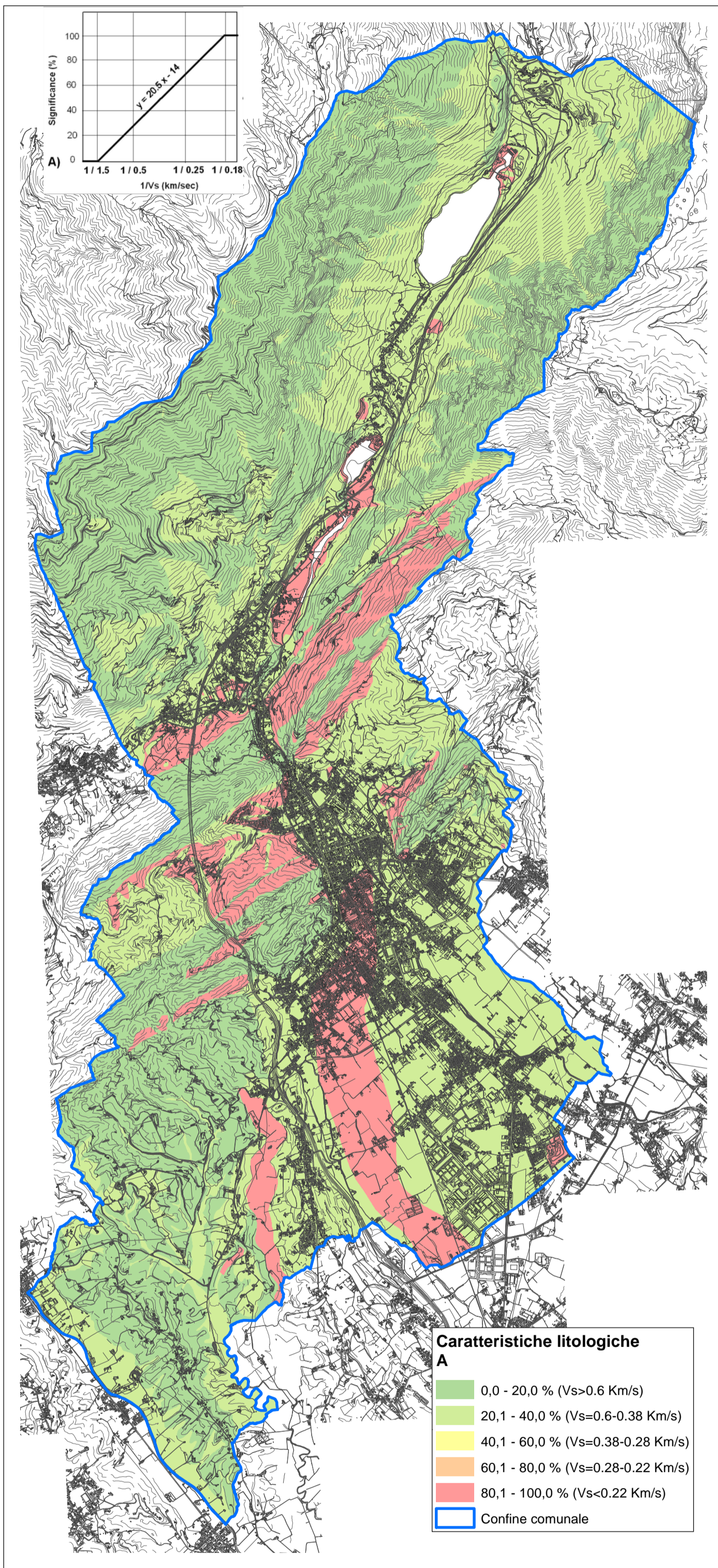
Parametro A: Litologia
