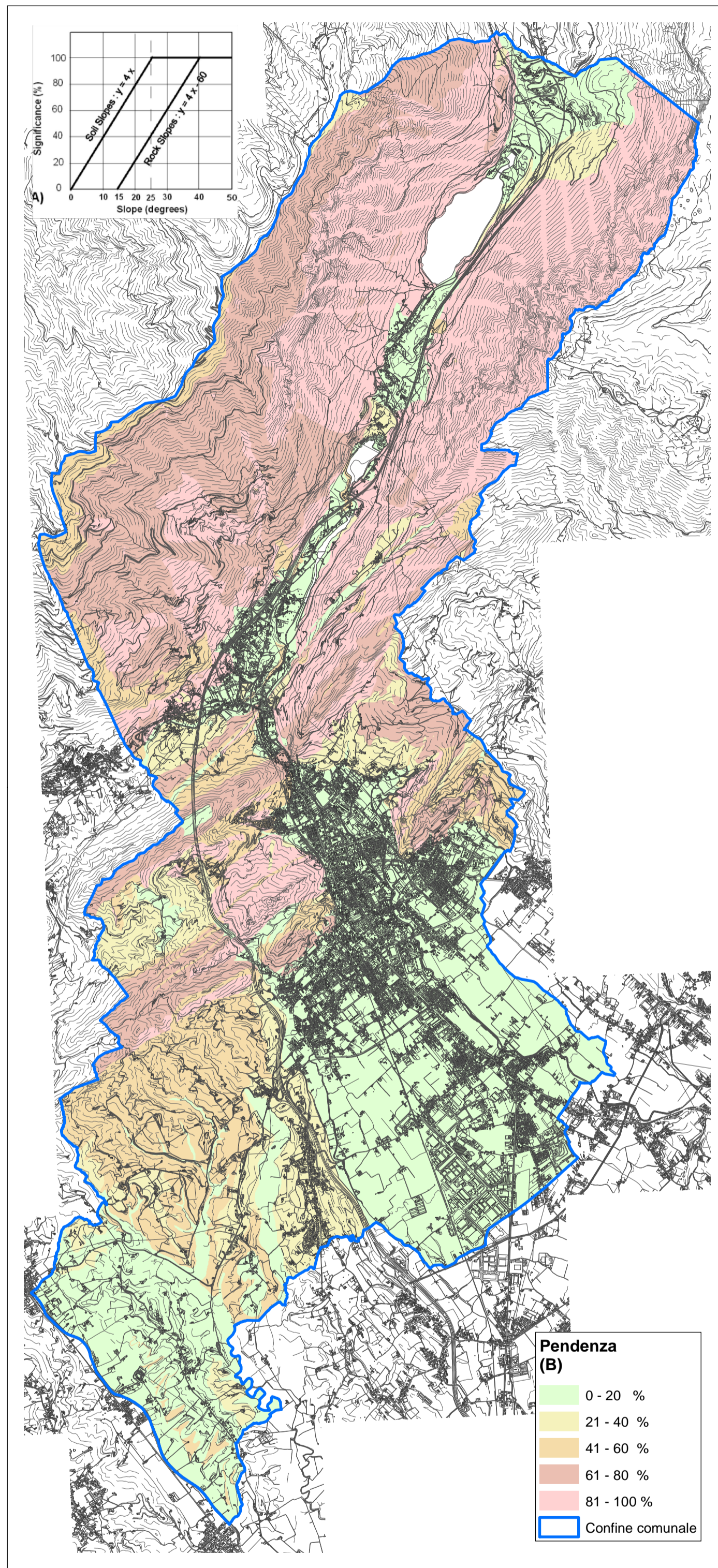
Parametro B: Pendenza
